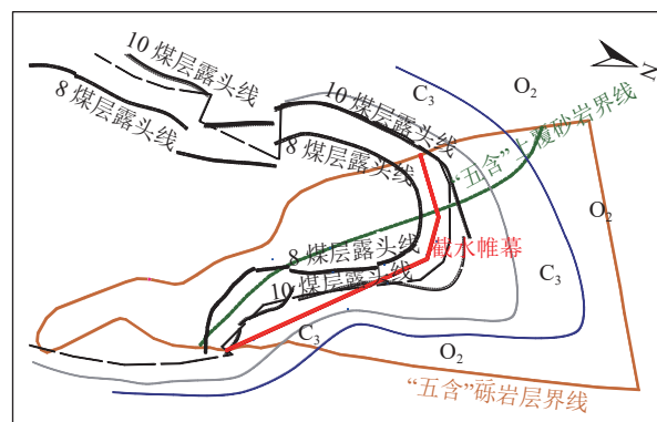
图2 朱仙庄煤矿帷幕平面示意
