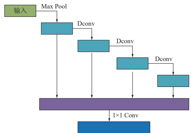
图 4 OSA 结构
