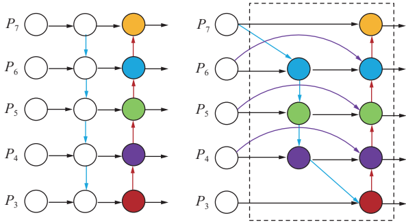
图 3 BiFPN 结构
