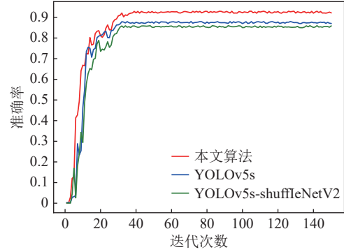
图 7 准确率曲线
