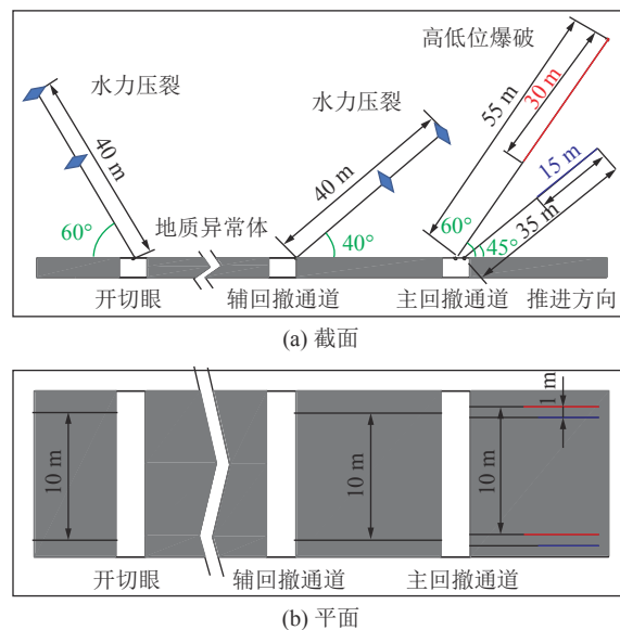
图 10 水力压裂与爆破切顶措施示意
