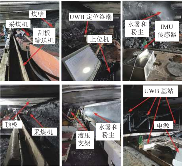
图 7 井下采煤机 IMU/UWB 融合定位现场试验场景
