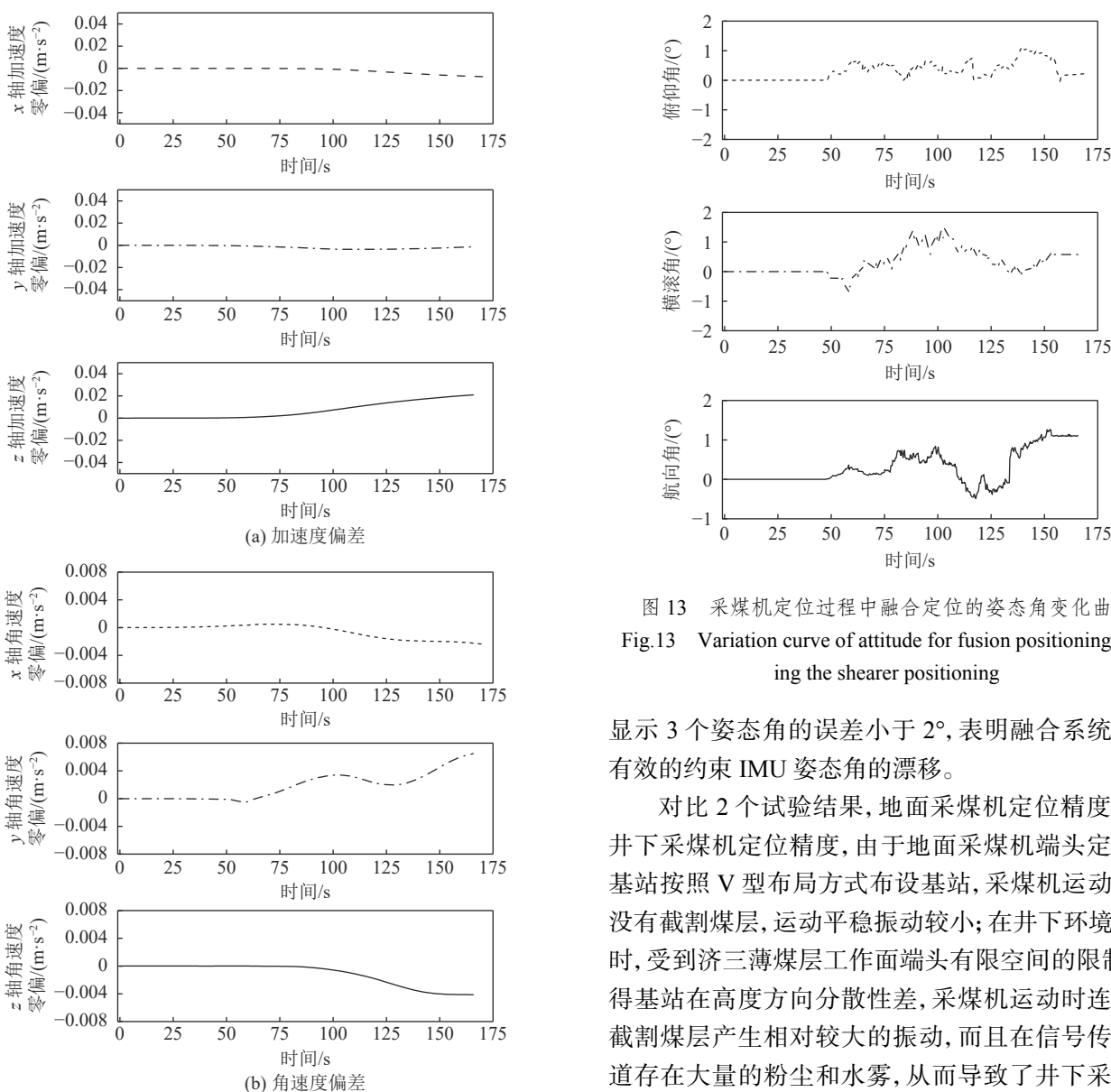
图 12 采煤机定位过程中 IMU 的加速度偏差和角速度偏差变化曲线
