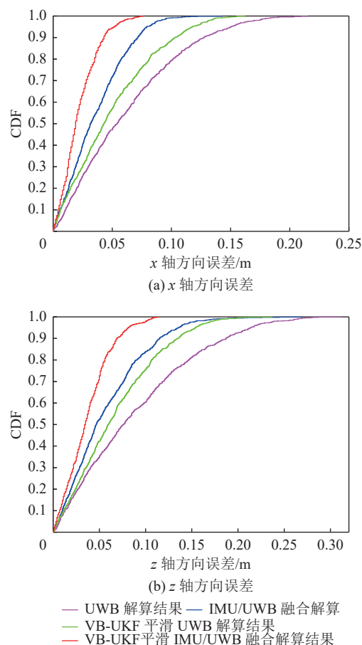
图 6 地面采煤机试验的 IMU/UWB 融合定位结果 x 轴和 z 轴方向定位误差的 CDF 曲线
