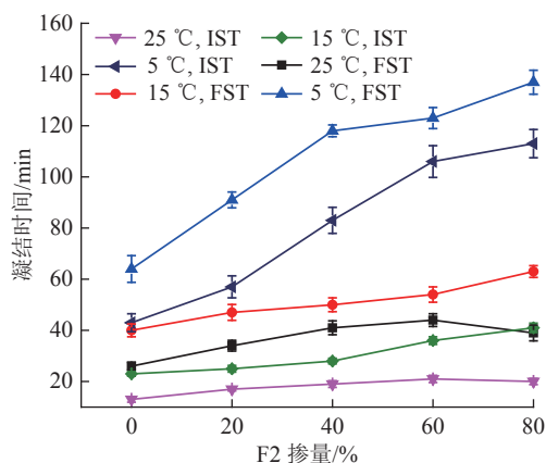
图10 F2掺量对高水充填材料凝结时间的影响
