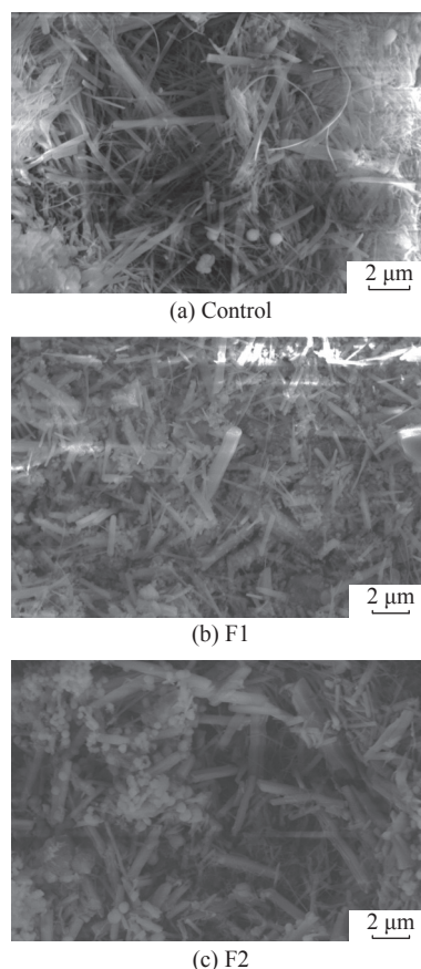
图 15 高水充填材料 28 d SEM
