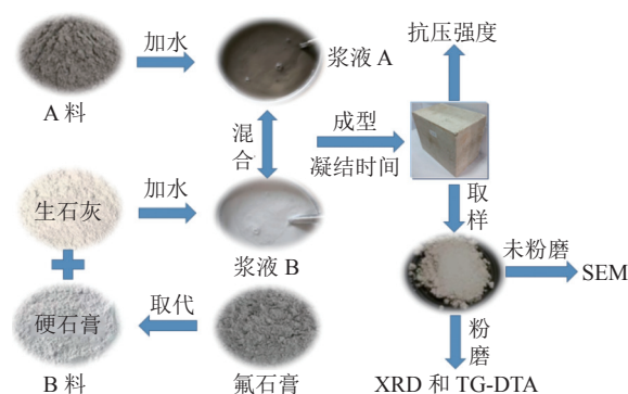
图 8 试验流程
