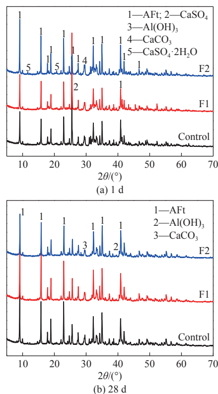
图13 高水充填材料的XRD图
