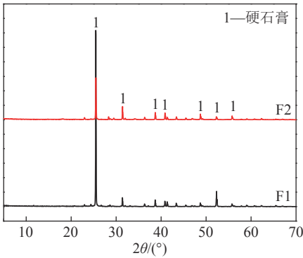
图 4 氟石膏的 XRD
