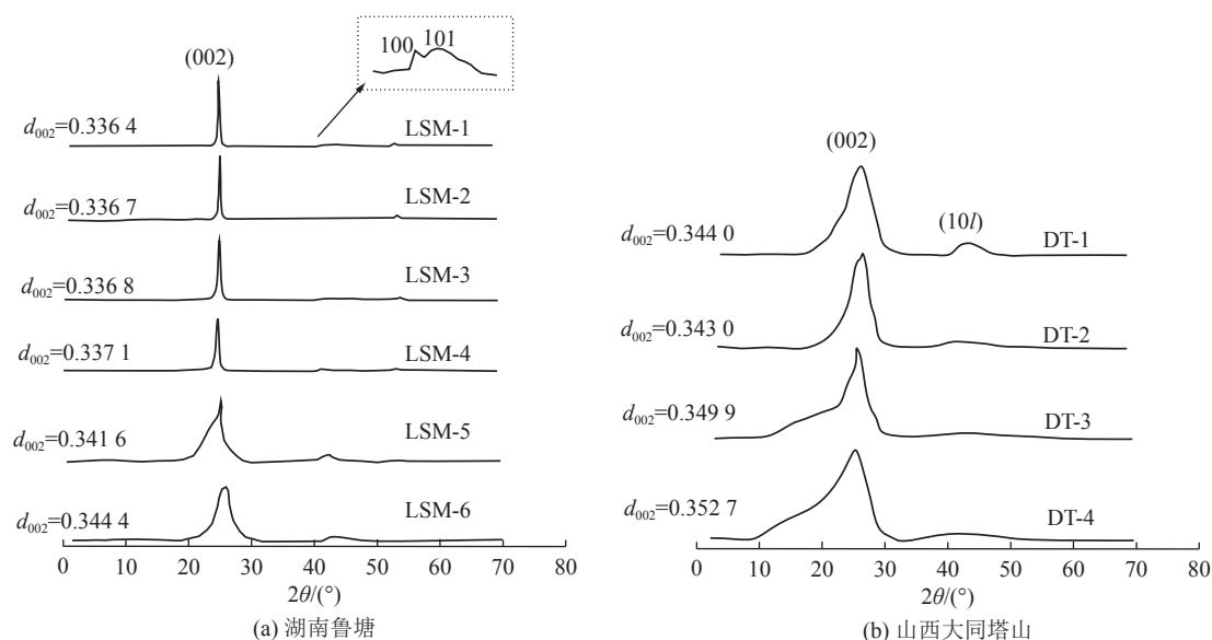
图 2 接触变质煤 XRD 图谱
