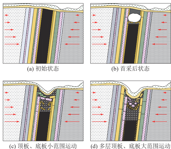
图 3 覆岩结构破断失稳演化过程
