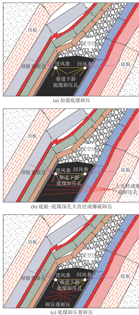
图 7 结合防突体系的卸压优化方案
