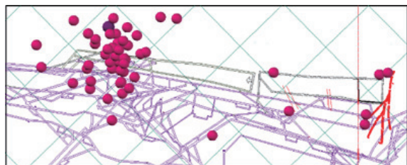
图9 5521-20工作面2016年12月微震事件分布 (大于 10^4 J)
