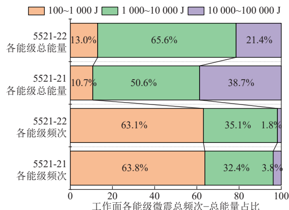
图 10 5521-22 和 5521-21 工作面同时间段各能级矿震总频次-总能量占比
