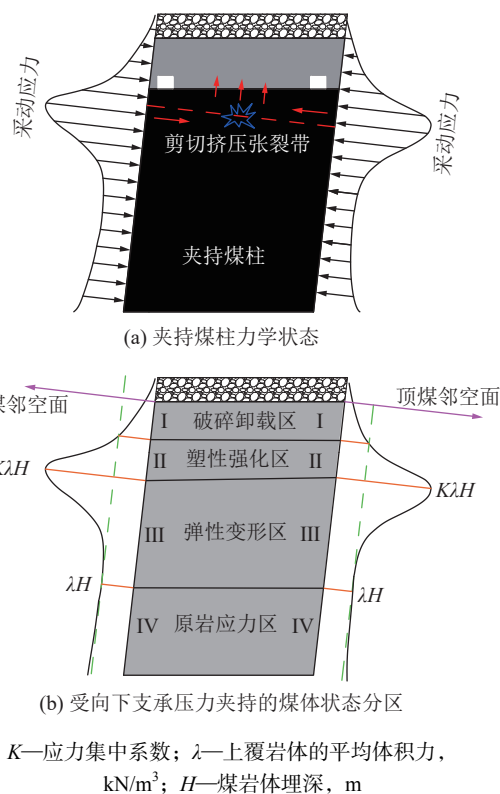
图 4 夹持煤柱力学状态分区 [32]
