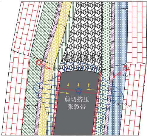
图 5 夹持煤柱型冲击机制
