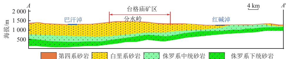
图 2 水文地质剖面图
