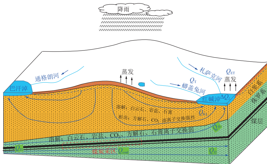
图 6 台格庙矿区地下水循环示意
