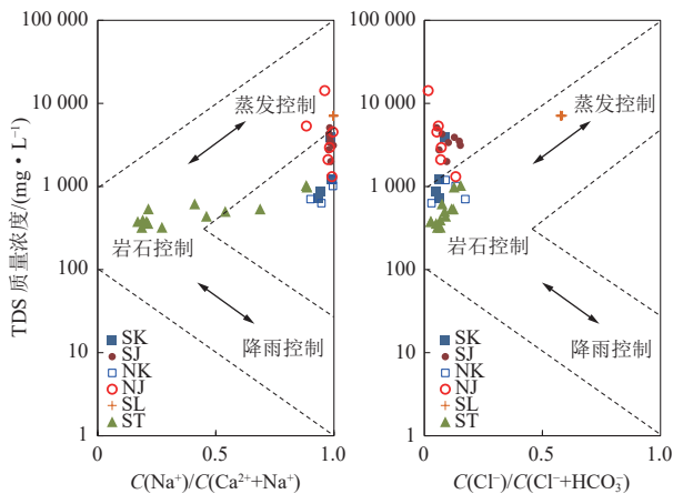
图 4 水化学 Gibbs 图
