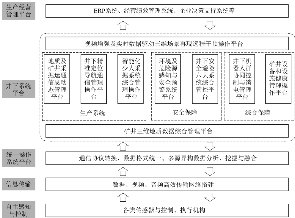
图 1 智能化煤矿技术架构
