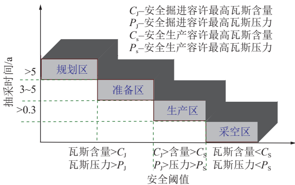
图2 煤与煤层气共采“四区”转换条件
