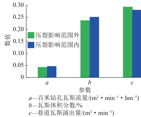
图 11 煤层压裂影响区内外煤层气抽采效果对比
