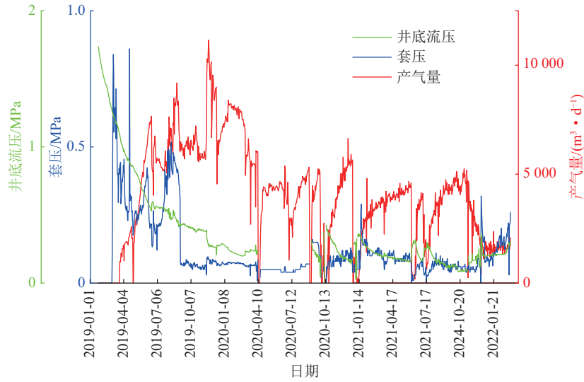
图 9 2017ZX-U-01 井生产数据
