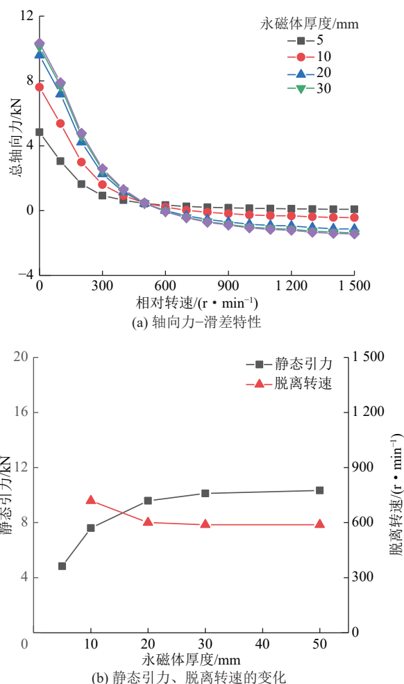
图13 永磁体厚度对轴向力-滑差特性的影响
