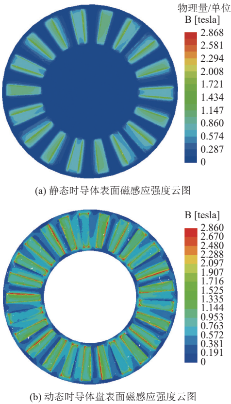
图 4 动态和静态时导体盘表面的磁感应强度云图
