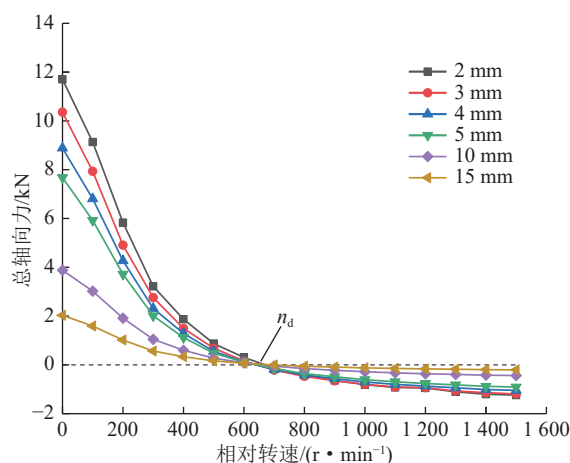
图9 气隙变化对轴向力特性的影响
