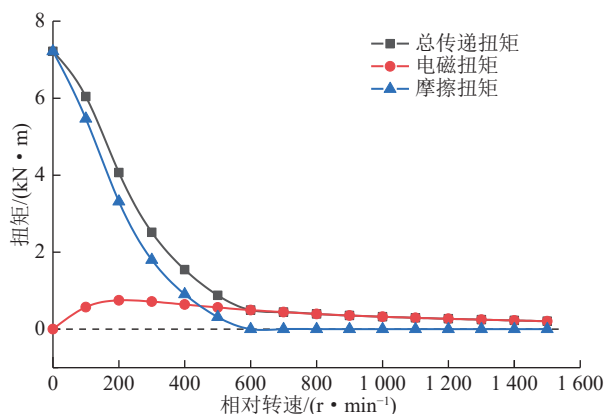
图8 永磁涡流限矩器的传递转矩特性
