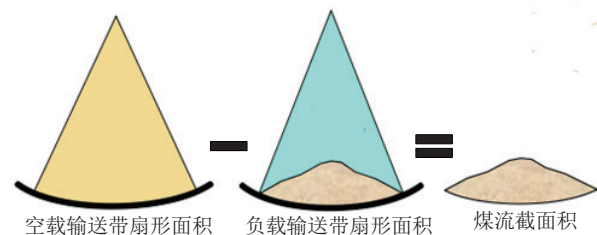
图10 激光雷达检测煤流量原理 [39]
