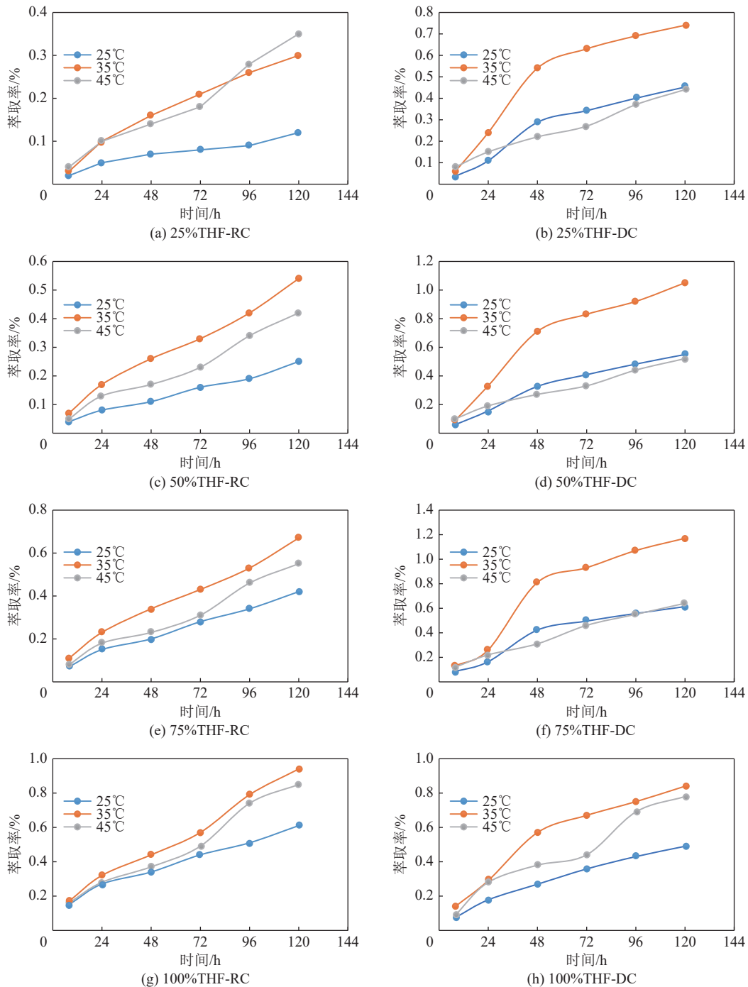
图4 不同温度下THF萃取酸化前后焦煤累计萃取率趋势
