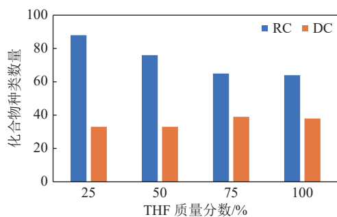
图5 RC及DC萃取物中化合物种类数量
