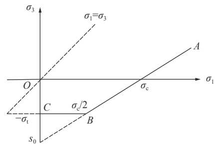
图 4 带有拉伸破坏的 Mohr-Coulomb 屈服准则强度包线
