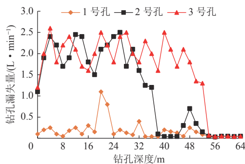
图10 钻孔1~3的钻孔深度与钻孔漏失量关系
