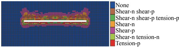
图 7 采场底板倾向塑性区分布
