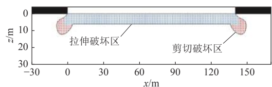
图 5 采场底板破坏形态
