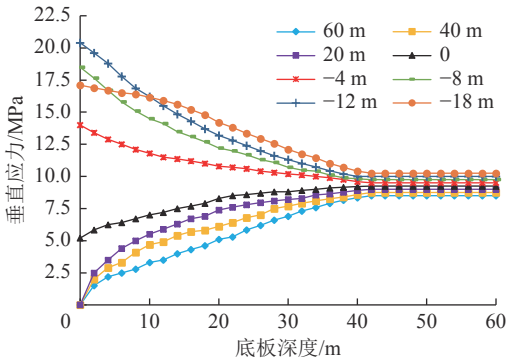
图 8 采场底板深度与垂直应力关系
