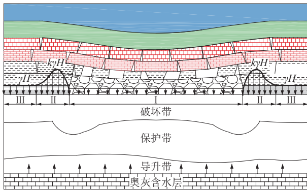
图2 承压水上采场底板沿工作面倾向受力示意图
