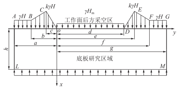
图3 采场底板倾向力学计算模型
