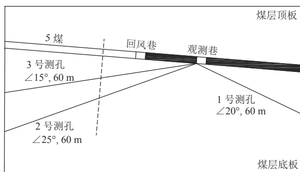
图9 钻孔布置剖面图
