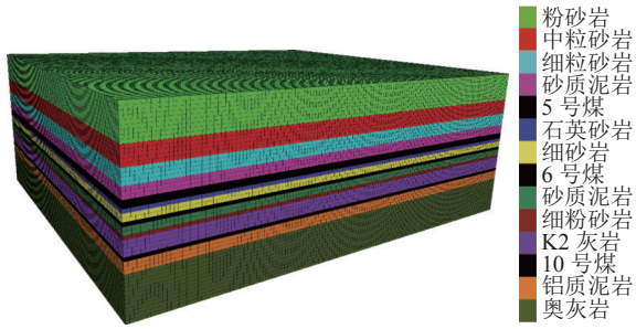
图 6 数值计算模型建立
