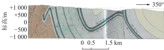
图 1 乌东矿区构造 [22]
