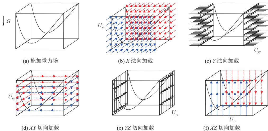
图 5 地应力反演单位加载步骤
