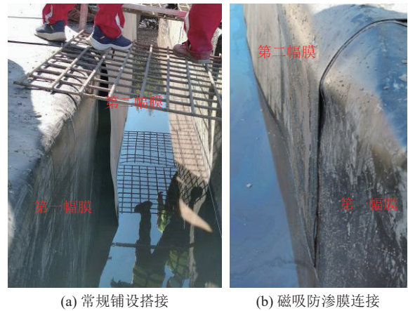
图 7 柔性磁吸防渗膜与常规铺设效果对比
