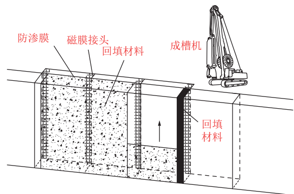
图 8 柔性磁吸防渗膜帷幕填充示意图
