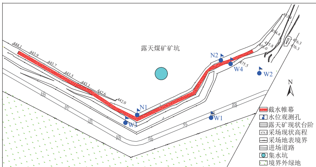
图4 试验区截水帷幕平面示意
